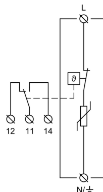
Schemat okablowania wewnętrznego
