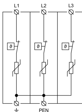
Schemat okablowania wewnętrznego
